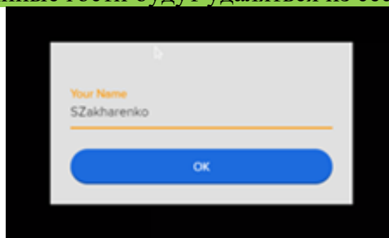
Рисунок 4. Ввод имени
